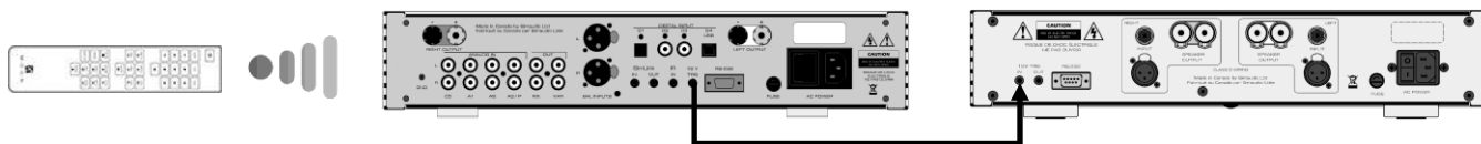
Figure 7: Commande à distance utilisant un Trigger 12V
