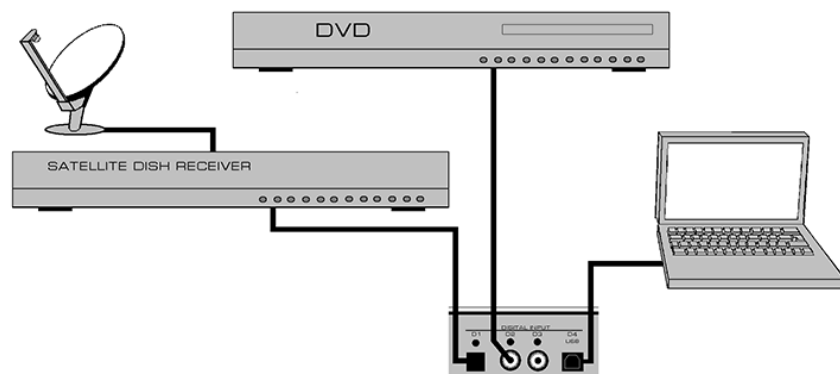
Figure 2: Entrées numériques en option du MOON 340i X – exemples de connexions
